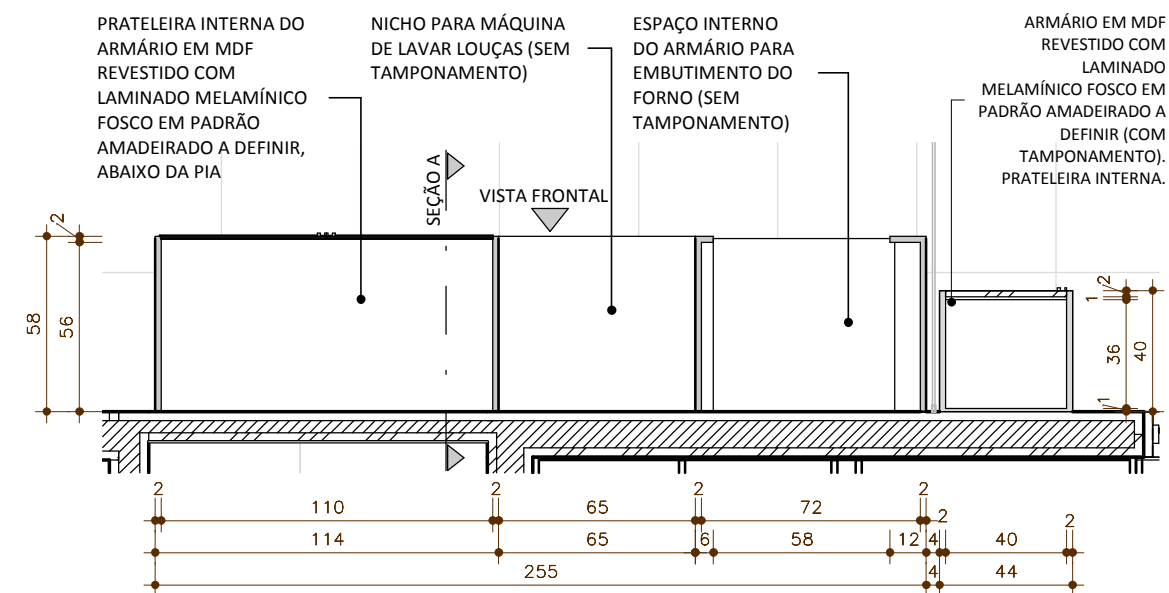
5 ARMÁRIOS DA BANCADA DA COZINHA - SEÇÃO HORIZONTAL B ESCALA 1 : 25
