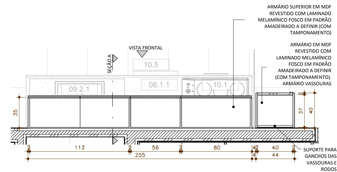
4 ARMÁRIOS DA BANCADA DA COZINHA - SEÇÃO HORIZONTAL A ESCALA 1 : 25
