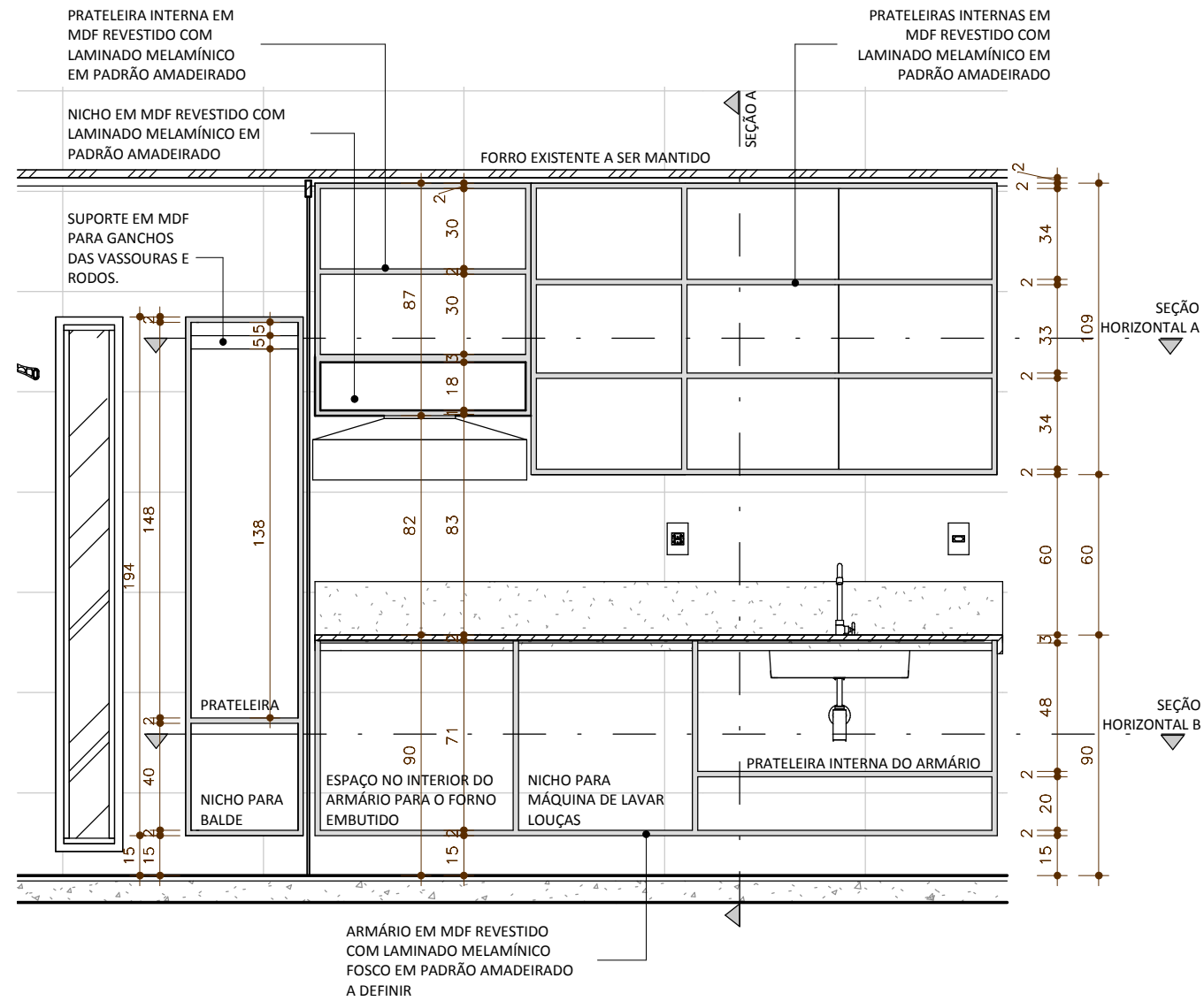
2 ARMÁRIO DA BANCADA DA COZINHA - VISTA FRONTAL INTERNA ESCALA 1 : 25
