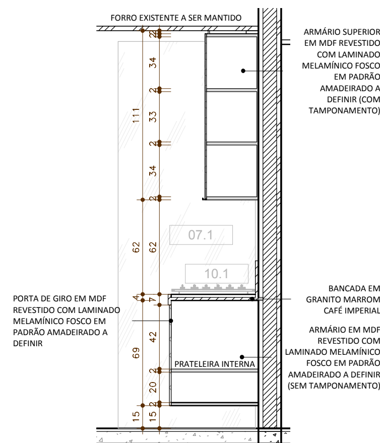
3 ARMÁRIO DA BANCADA DA COZINHA - SEÇÃO VERTICAL A ESCALA 1 : 25
