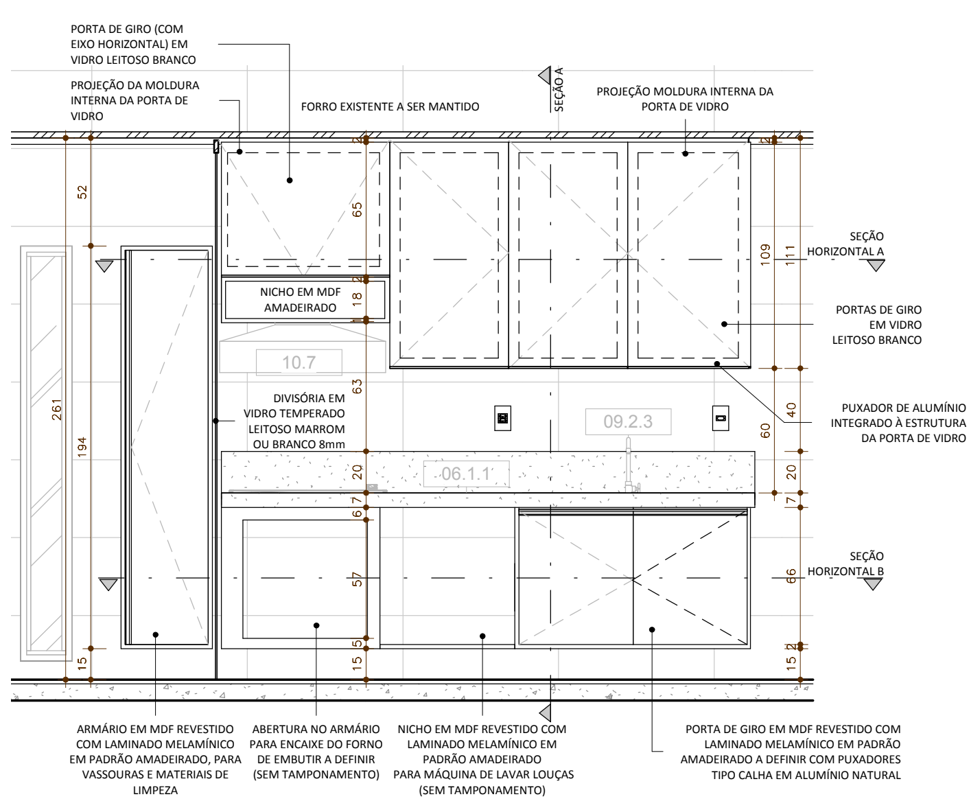
1 ARMÁRIO DA BANCADA DA COZINHA E ÁREA DE SERVIÇO - VISTA FRONTAL EXTERNA ESCALA 1 : 25
