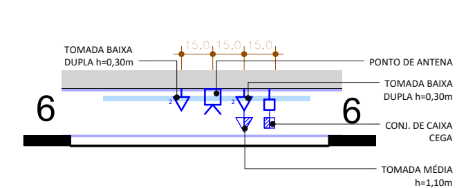
7. DET. ELÉTRICA - SUÍTE PIETRA ESCALA 1:25
