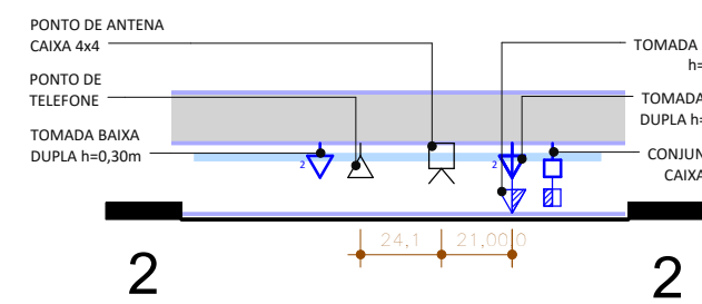
3. DET. ELÉTRICA - SALA ESCALA 1:25
