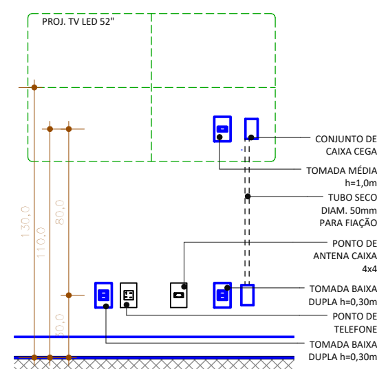
2. VISTA ELÉTRICA - SALA ESCALA 1:25
