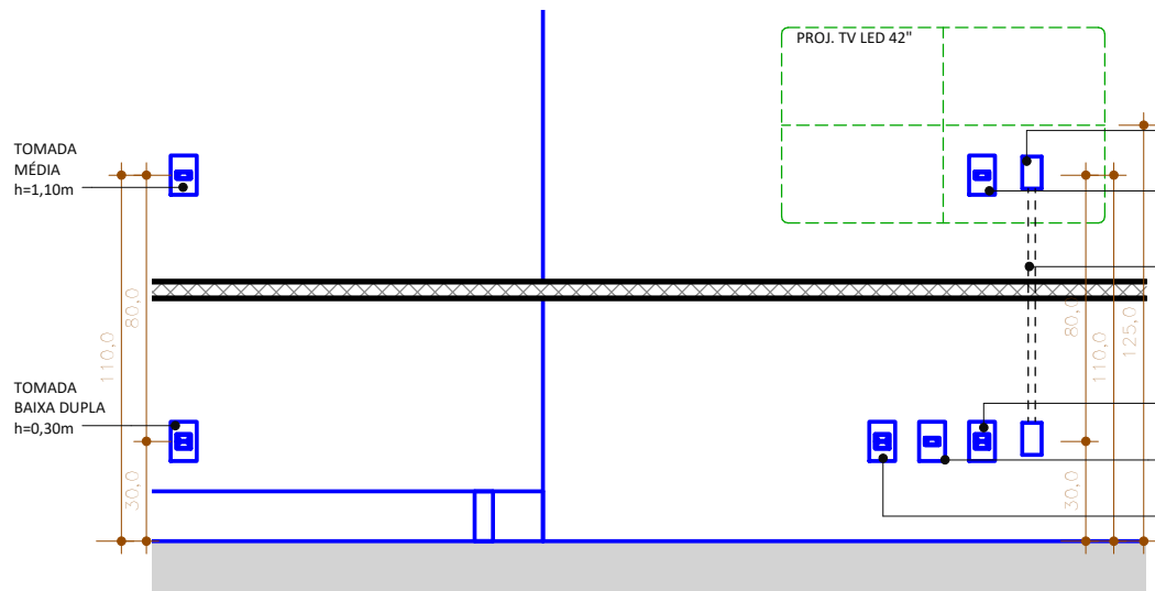
4. VISTA ELÉTRICA - SUÍTE RUY ESCALA 1:25
