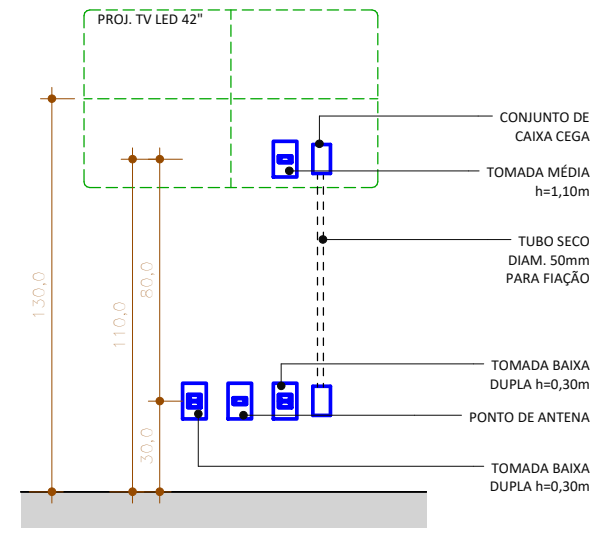
6. VISTA ELÉTRICA - SUÍTE PIETRA ESCALA 1:25
