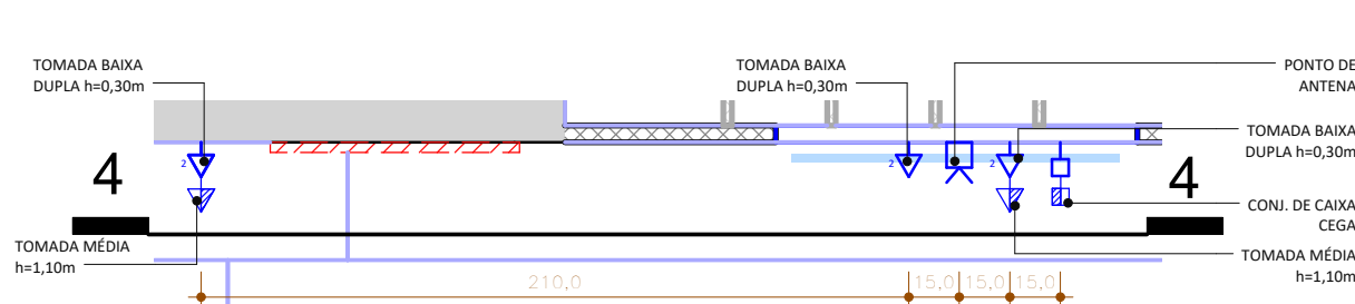
5. DET. ELÉTRICA - SUÍTE RUY ESCALA 1:25
