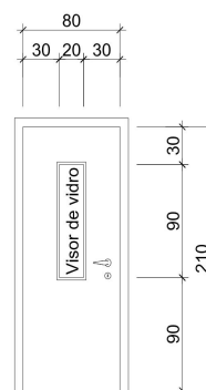
Figura 2: Desenho esquemático da porta com visor de vidro.
